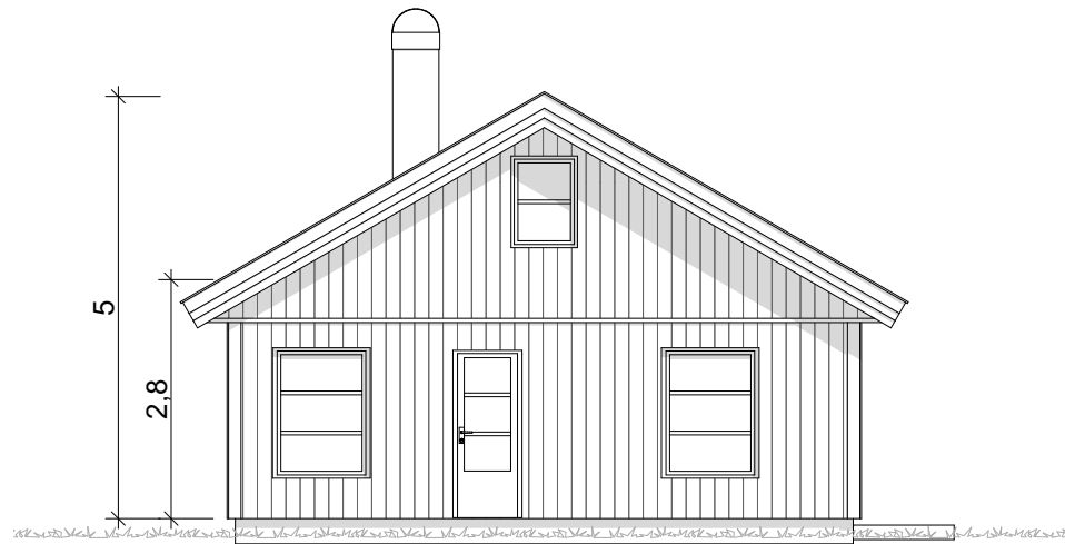
Fasade 2
