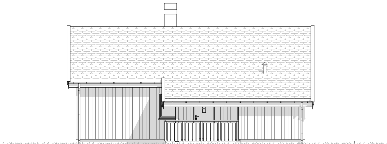
Fasade 1
