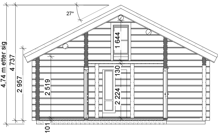
Snitt A-A
